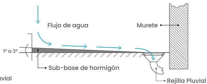
ESCURRIMIENTO PLUVIAL CON MURETE
